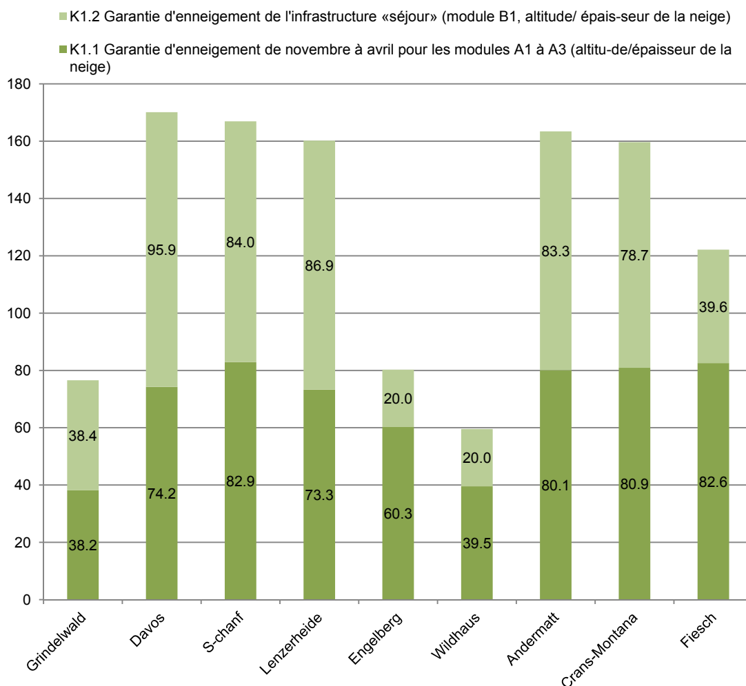
Figure 3: Evaluation des critères de l'objectif K1: «Garantie d'enneigement des installations de sports de neige et de l'infrastructure «séjour» du centre»
